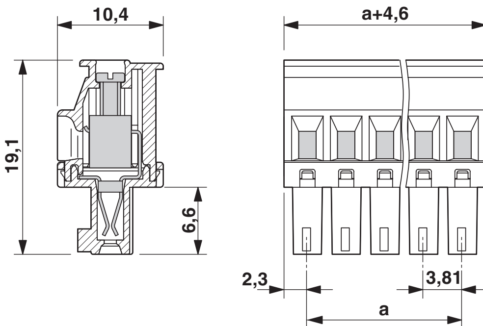
Rysunek wymiarowy
