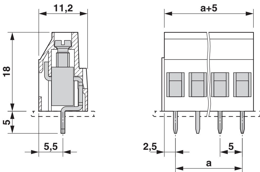
Rysunek wymiarowy
