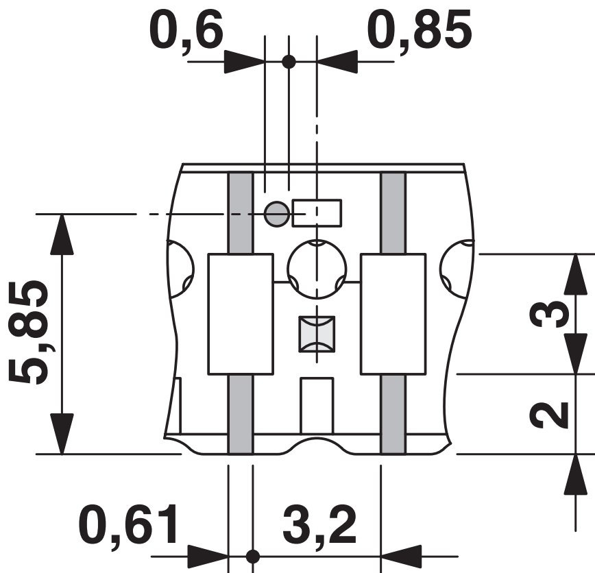
Rysunek wymiarowy
