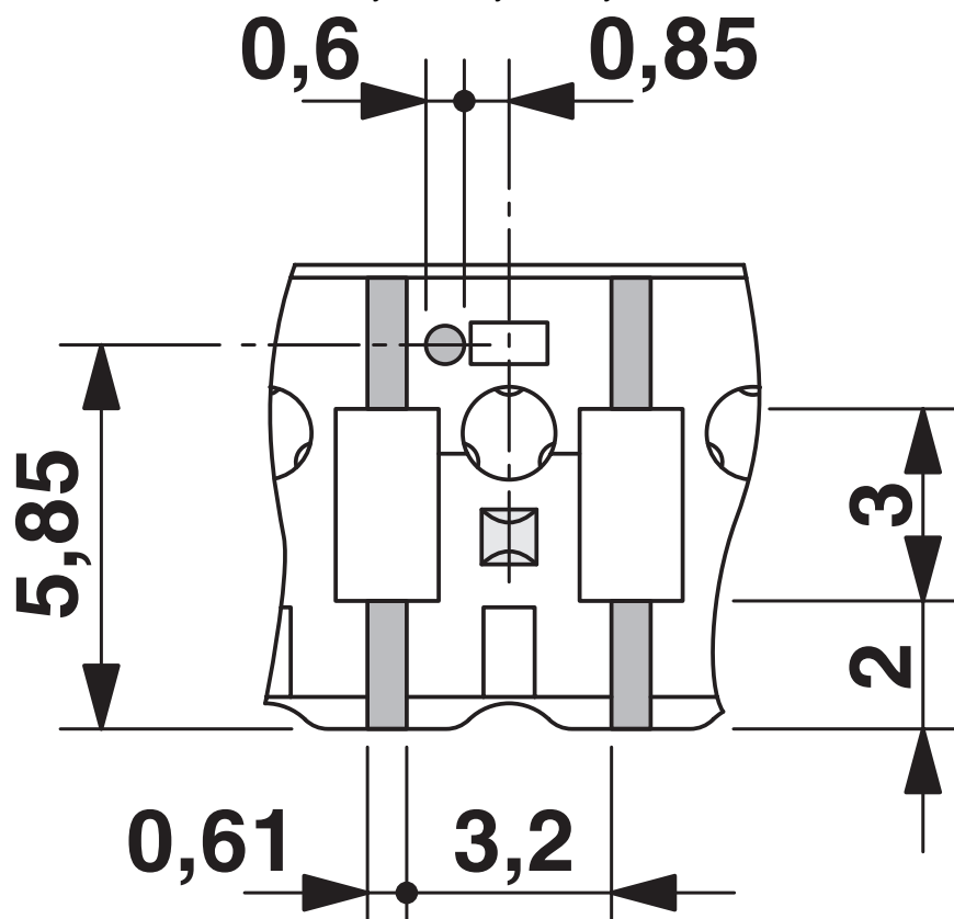
Rysunek wymiarowy
