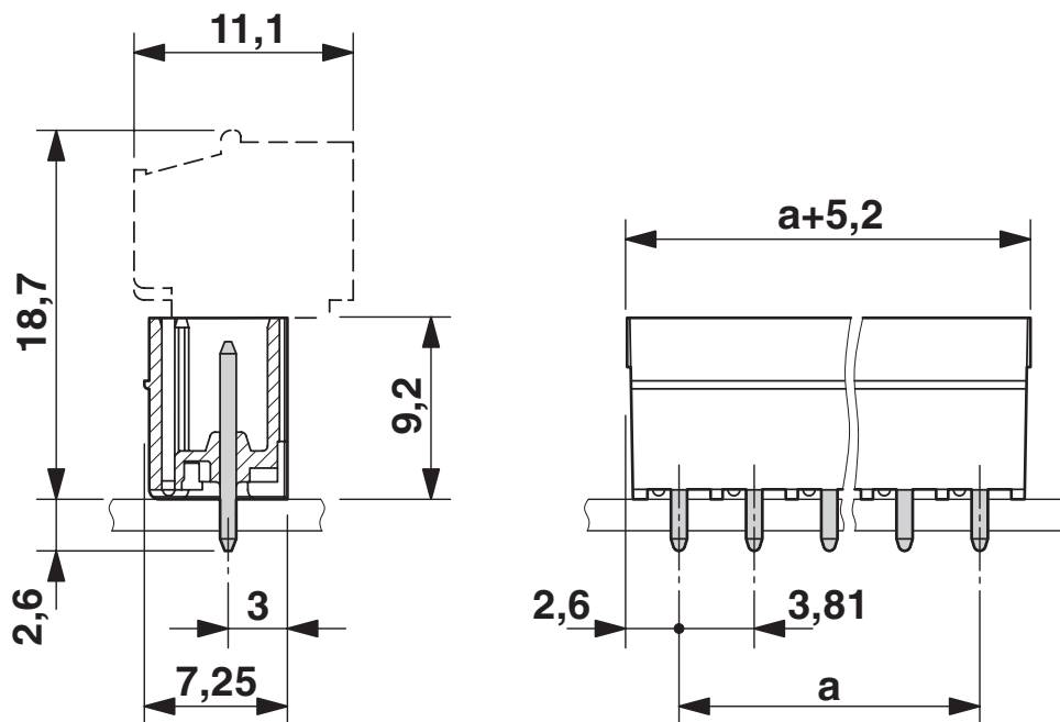
Rysunek wymiarowy
