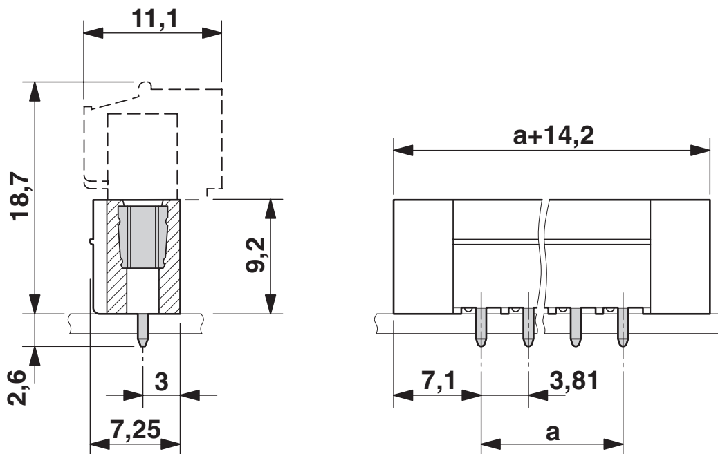
Rysunek wymiarowy
