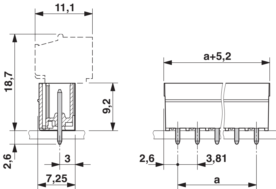
Rysunek wymiarowy
