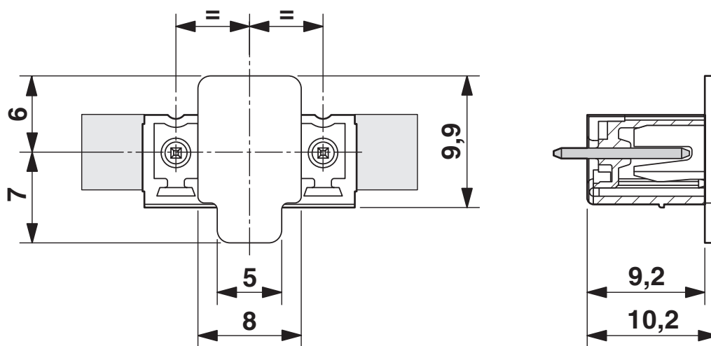
Rysunek wymiarowy
