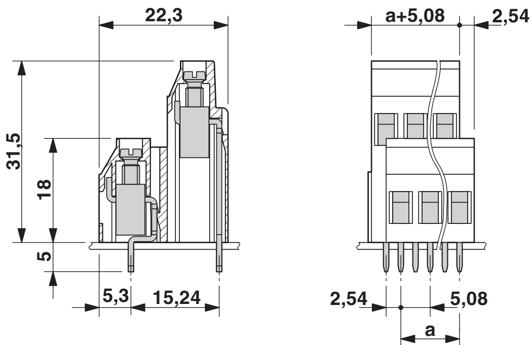
Rysunek wymiarowy
