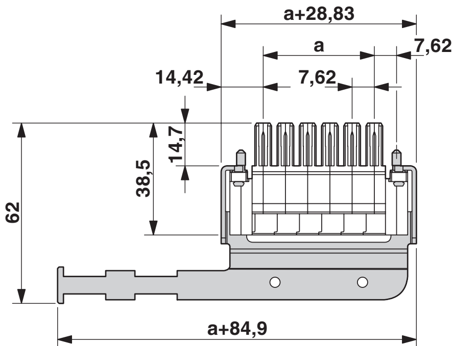
Rysunek wymiarowy
