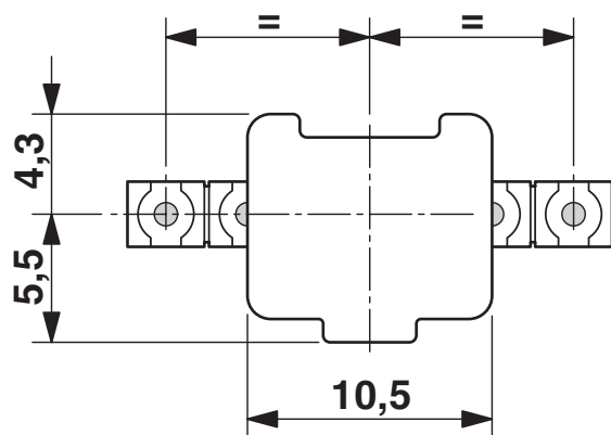
Rysunek wymiarowy
