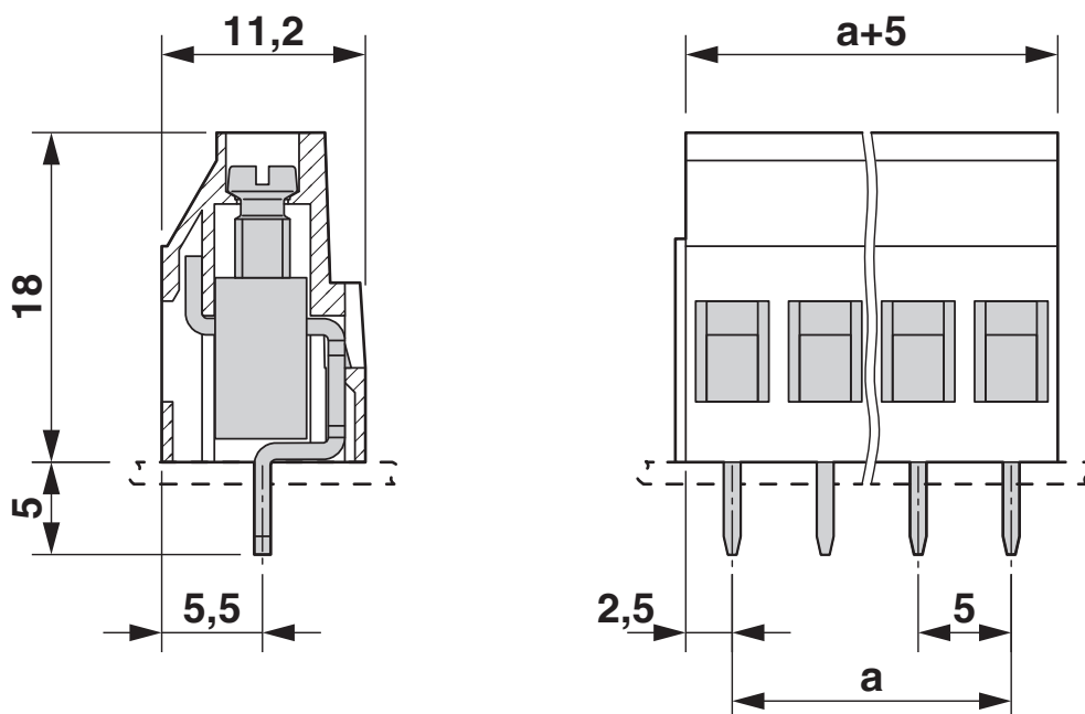
Rysunek wymiarowy
