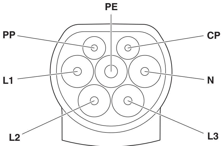
rysunek złączy
