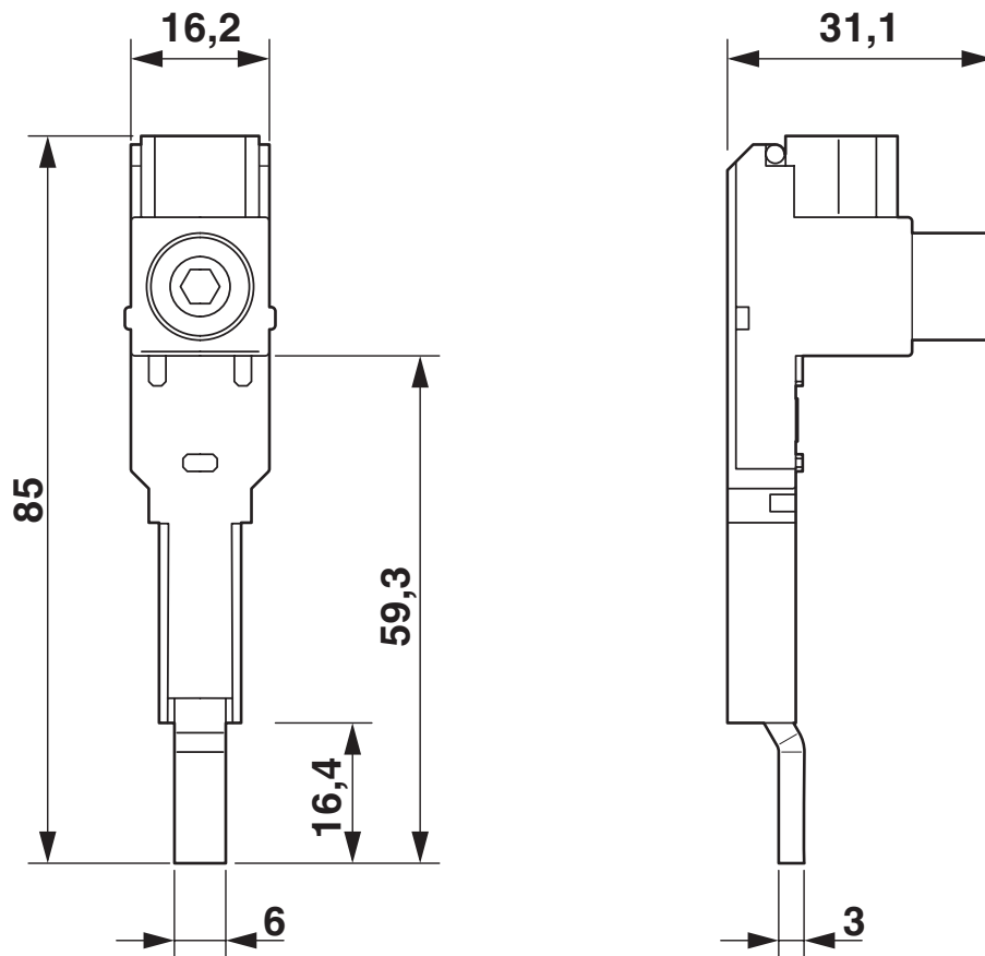
Rysunek wymiarowy
