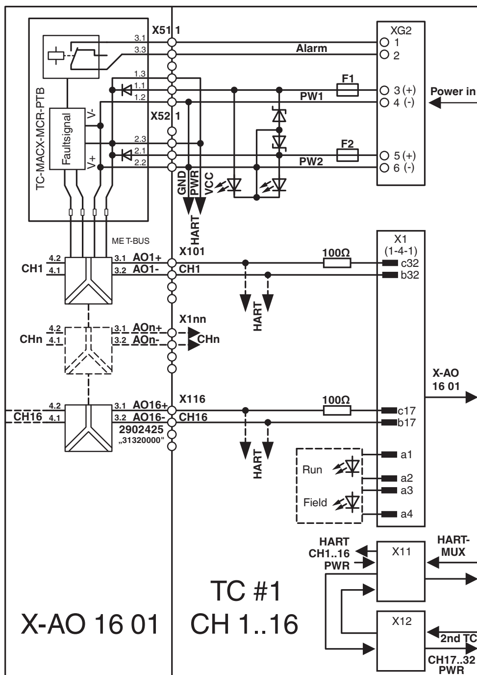
Schemat blokowy
