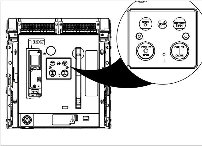
Figure 27. Step 3.
